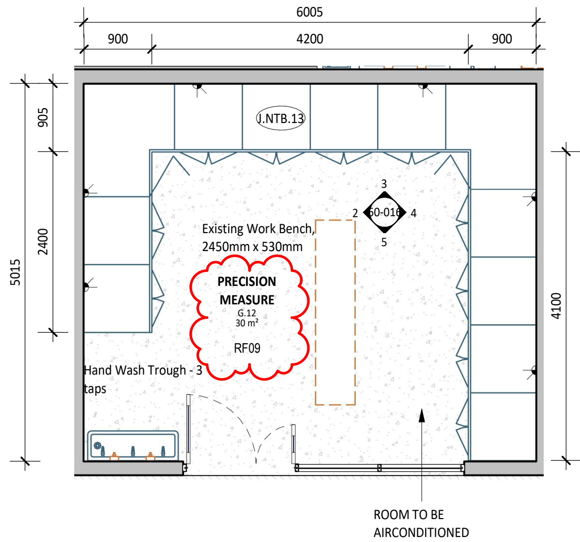
1 PLAN DETAIL 30-01 1 : 50
